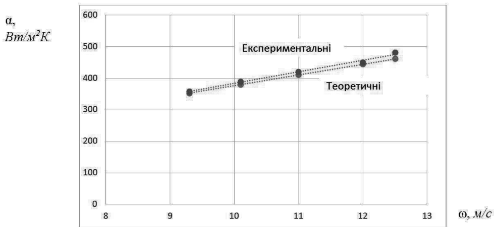
Рис. 7. Залежність коефіцієнта тепловіддачі від швидкості потоку теплоносія, розраховані за модифікованим критеріальним рівнянням.
