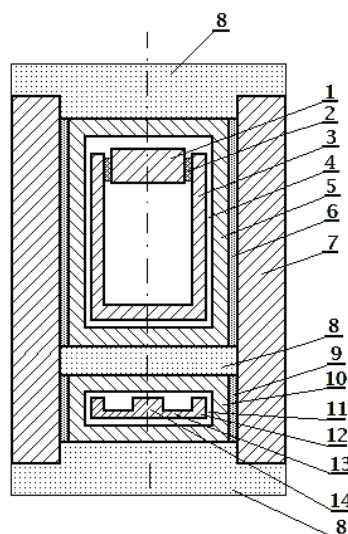
Рис. 1. Спрощена модель теплового блоку квазидиференціального калориметра.
