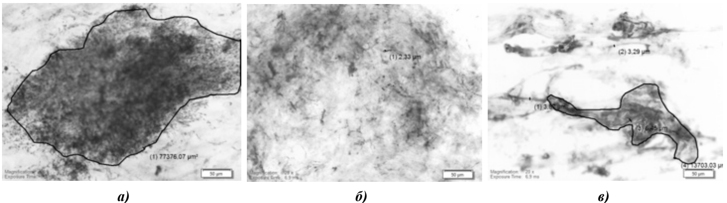
Рис. 4. Мікроструктура грибною суспензії, отриманої після ДІВЕ-обробки плодового тіла гриба шийтаке в РПА двох варіантів компоновки робочих органів: а, б) 1-й варіант: ротор-статор-ротор; в) 2-й варіант: статор-ротор-статор.
